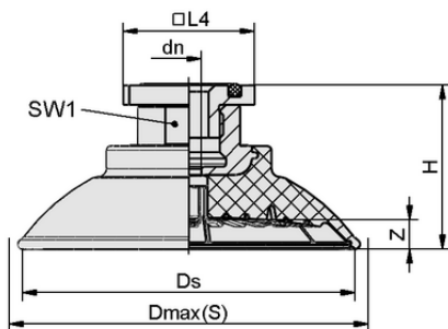
Datos de diseño SAF 60 NBR-60 RA
