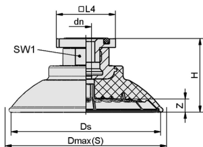
Конструктивные данные SAF 50 NBR-60 RA
