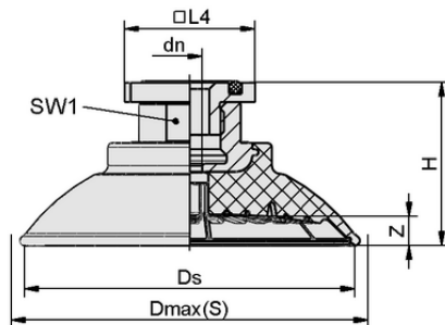
Données de construction SAF 50 NBR-60 RA
