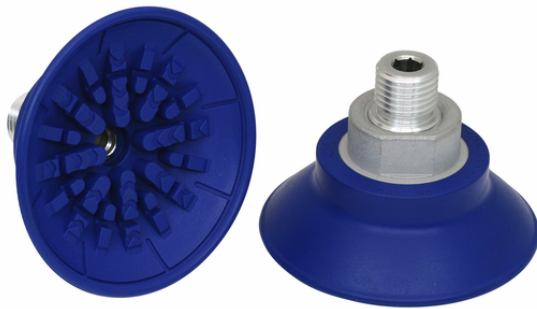
SAF 60 NBR-60 M14x1.5-AG
