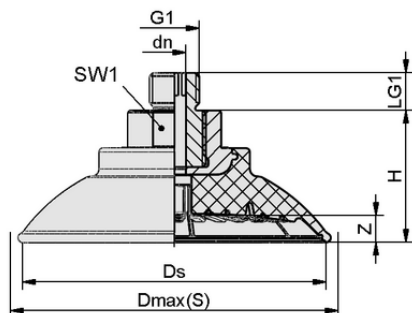
Конструктивные данные SAF 30 NBR-60 M14x1.5-AG
