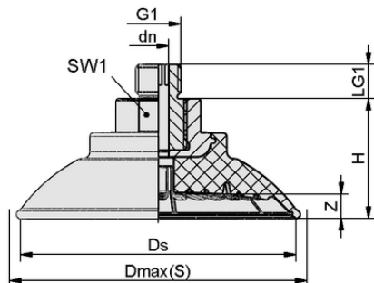
Dati di costruzione SAF 30 NBR-60 M10-AG
