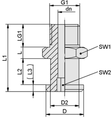
Tasarım verileri SA-NIP N012 G1/4-AG DN500
