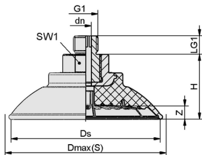
Конструктивные данные SAF 50 NBR-60 G1/4-AG
