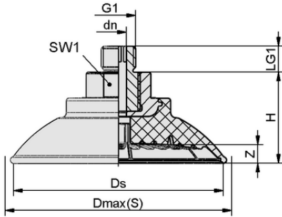
Tasarım verileri SAF 100 NBR-60 G1/4-AG
