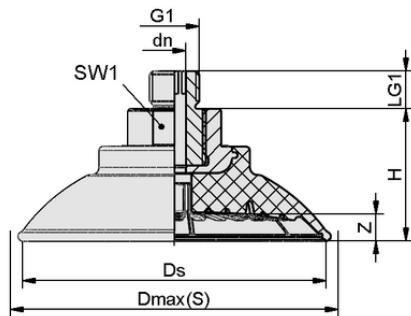
デザインデータ SAF 80 NBR-60 G1/4-AG
