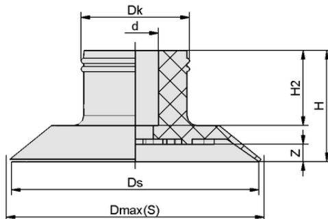
Конструктивные данные SGP 24 SI-50 N016
