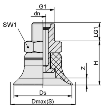
Конструктивные данные PFYN 50 NBR-CO-55 G1/8-AG
