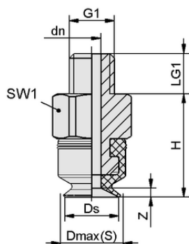
Конструктивные данные PFYN 8 NBR-CO-55 M5-AG
