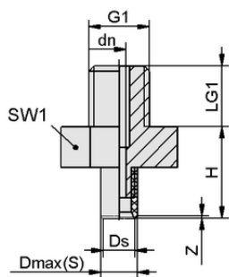
Конструктивные данные PFYN 1 NBR-CO-55 M3-AG
