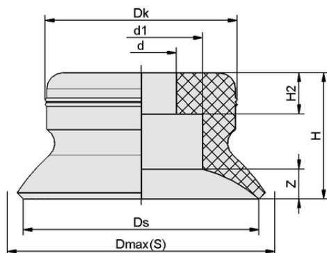
Dati di costruzione PFG 25 NBR-CO-55 N007
