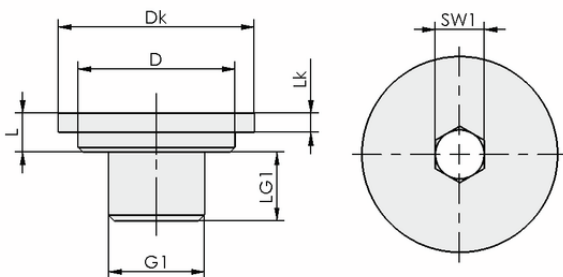
デザインデータ VRS-AN G1/4-AG
