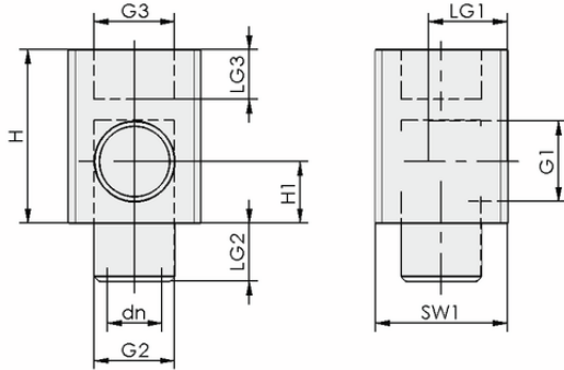
Tasarım verileri ANW G1/8-IG G1/8-AG
