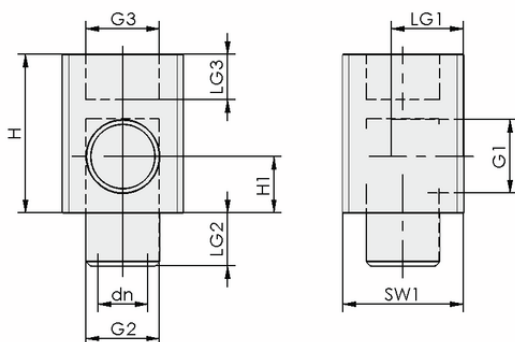
Конструктивные данные ANW G1/8-IG G1/8-AG
