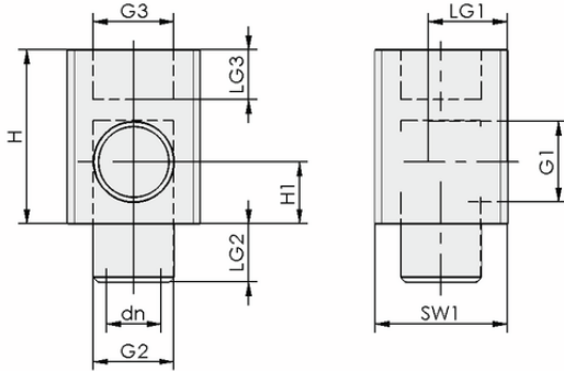
Tasarım verileri ANW G3/8-IG G1/2-AG
