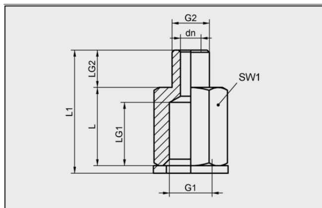
Конструктивные данные SA-NIP N009 G1/4-IG
