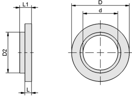
Tasarım verileri SCHE 38-21.5x5 ST VZ
