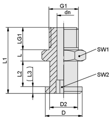
Конструктивные данные SA-NIP N005 G1/8-AG DN200
