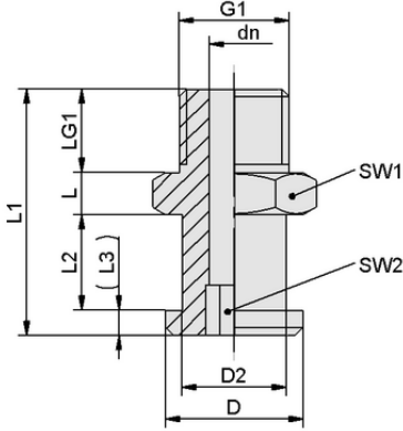
Tasarım verileri SA-NIP N004 G1/8-AG DN200
