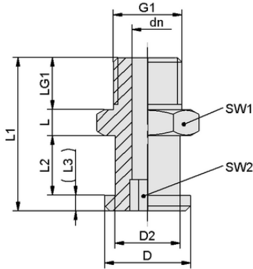
Tasarım verileri SA-NIP N004 M5-AG DN200
