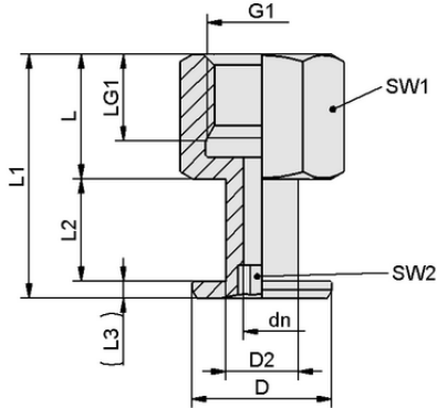
Tasarım verileri SA-NIP N008 G1/8-IG DN350
