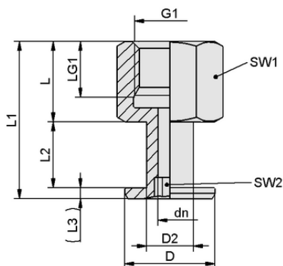
Données de construction SA-NIP N004 M5-IG DN200
