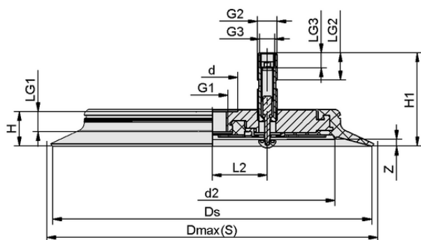
デザインデータ SPU 250 SI-60 G1/2-IG TV
