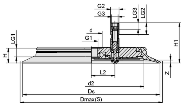
Конструктивные данные SPU 250 NBR-55 G1/2-IG TV
