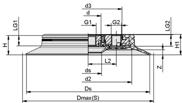
Конструктивные данные SPC 250 NBR-55 G1/2-IG
