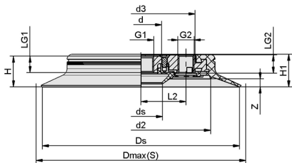
デザインデータ SPC 210 NBR-55 G1/2-IG
