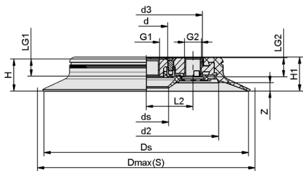
Конструктивные данные SPC 210 NBR-55 G1/2-IG
