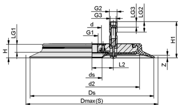
デザインデータ SPC 160 NBR-55 G1/2-IG TV
