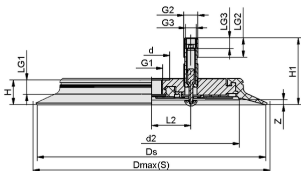
Конструктивные данные SPU 210 SI-60 G1/2-IG TV
