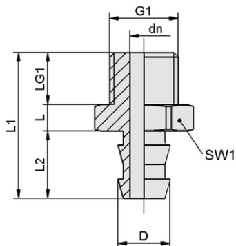
デザインデータ SA-NIP N035 G1/4-AG DN550
