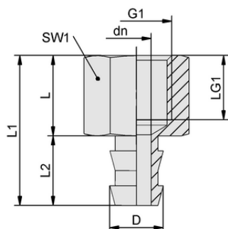
Конструктивные данные SA-NIP N035 G1/4-IG DN550
