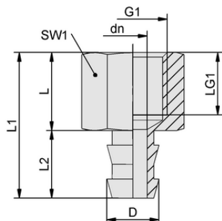
デザインデータ SA-NIP N035 G1/4-IG DN550
