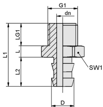
Dati di costruzione SA-NIP N034 G1/4-AG DN550
