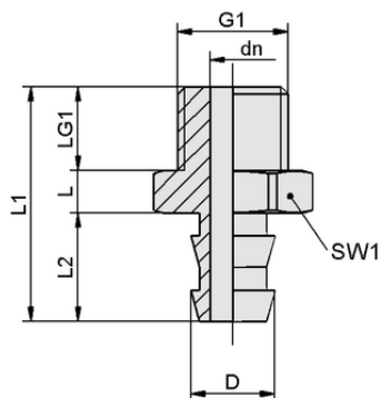
Datos de diseño SA-NIP N034 G1/4-AG DN550
