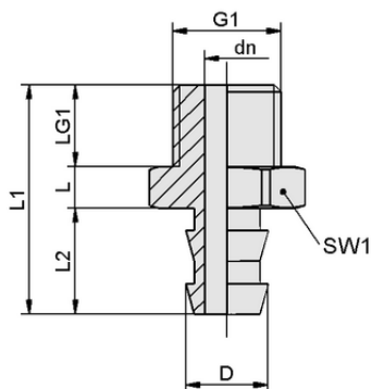
デザインデータ SA-NIP N034 G1/4-AG DN550
