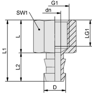
Tasarım verileri SA-NIP N034 G1/4-IG DN550
