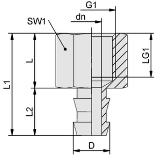
Tasarım verileri SA-NIP N033 G1/4-IG DN550
