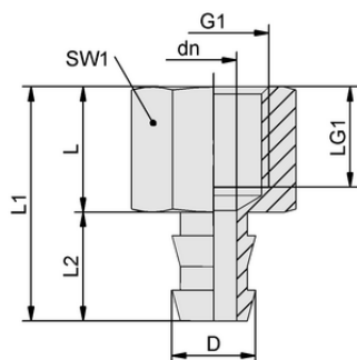
Dati di costruzione SA-NIP N033 G1/4-IG DN550
