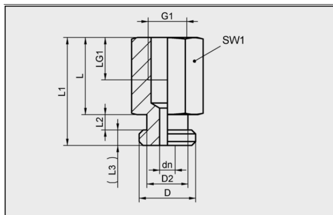
Données de construction SA-NIP N029 G1/8-IG DN350
