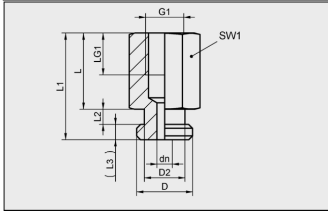
Tasarım verileri SA-NIP N029 G1/8-IG DN350
