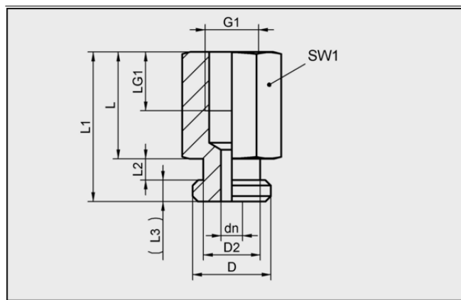
Datos de diseño SA-NIP N028 M5-IG DN200
