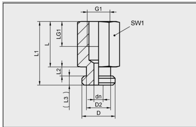
デザインデータ SA-NIP N028 M5-IG DN200
