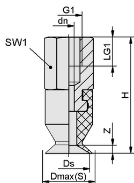
Конструктивные данные SGAN 13 PU-60 G1/8-IG
