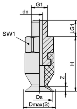
Dati di costruzione SGAN 13 SI-55 G1/8-AG
