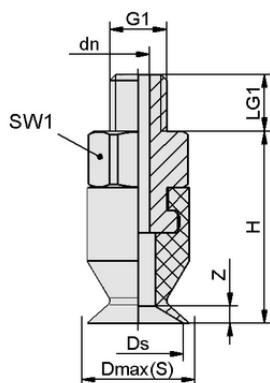
デザインデータ SGAN 13 SI-55 G1/8-AG
