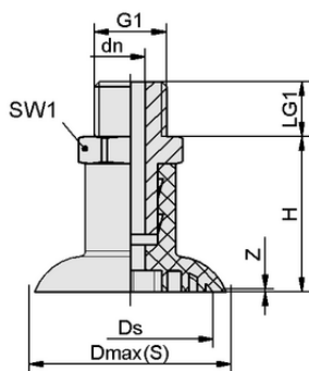
Datos de diseño SGPN 35 NK-40 G1/4-AG
